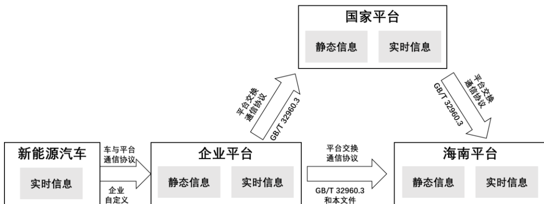
图 1 海南省新能源汽车公共数据采集架构
